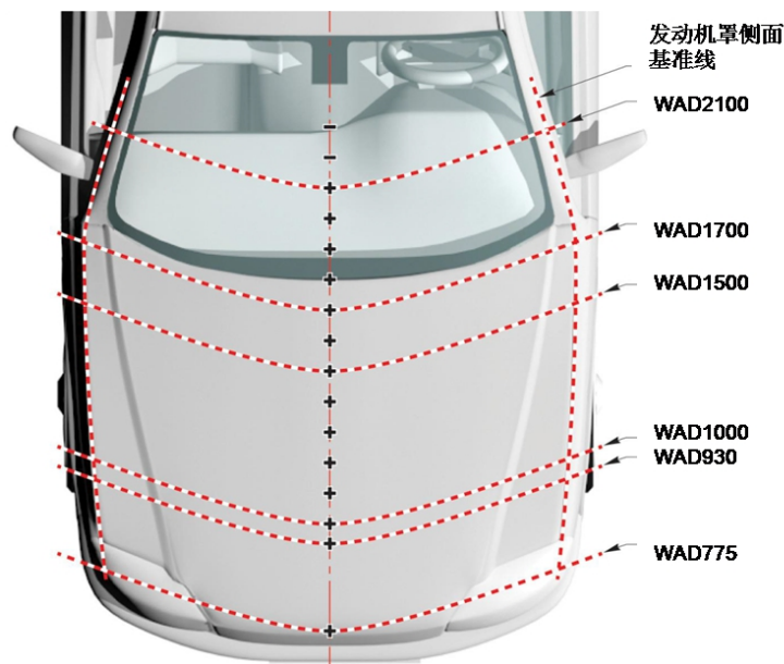
图 6 头型试验区域
