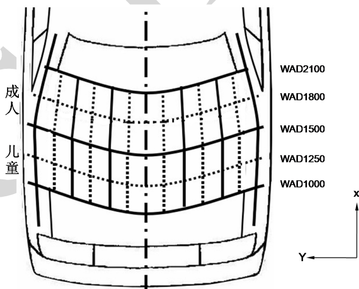
图 18 头型区域 12 等分
