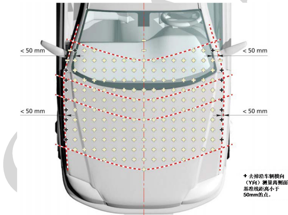
图 15 删除的网格点
