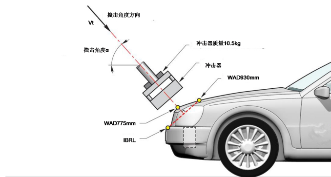
图 27 上腿型冲击 WAD775 试验
