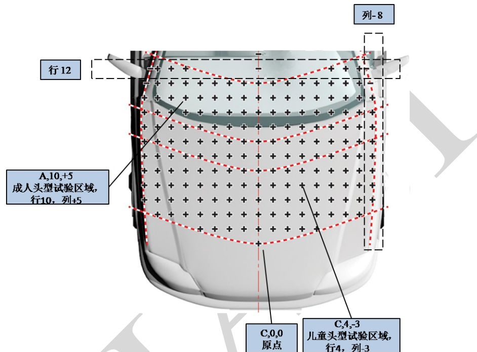
图 16 头型试验区域网格点的编号示例
