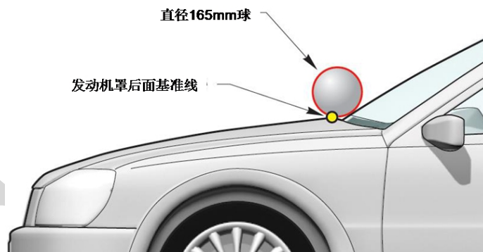
图 3 发动机罩后面基准线的确定
