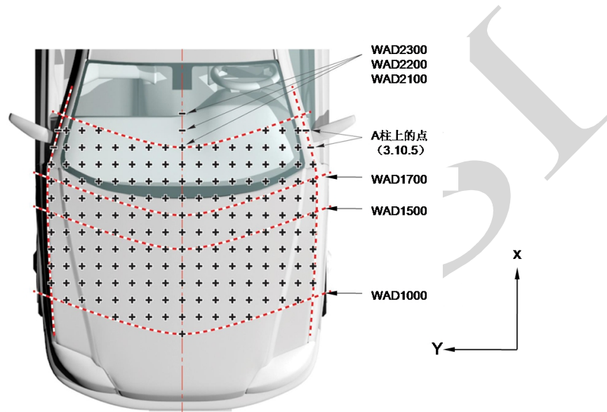
图 13 头型试验区域网格点标记
