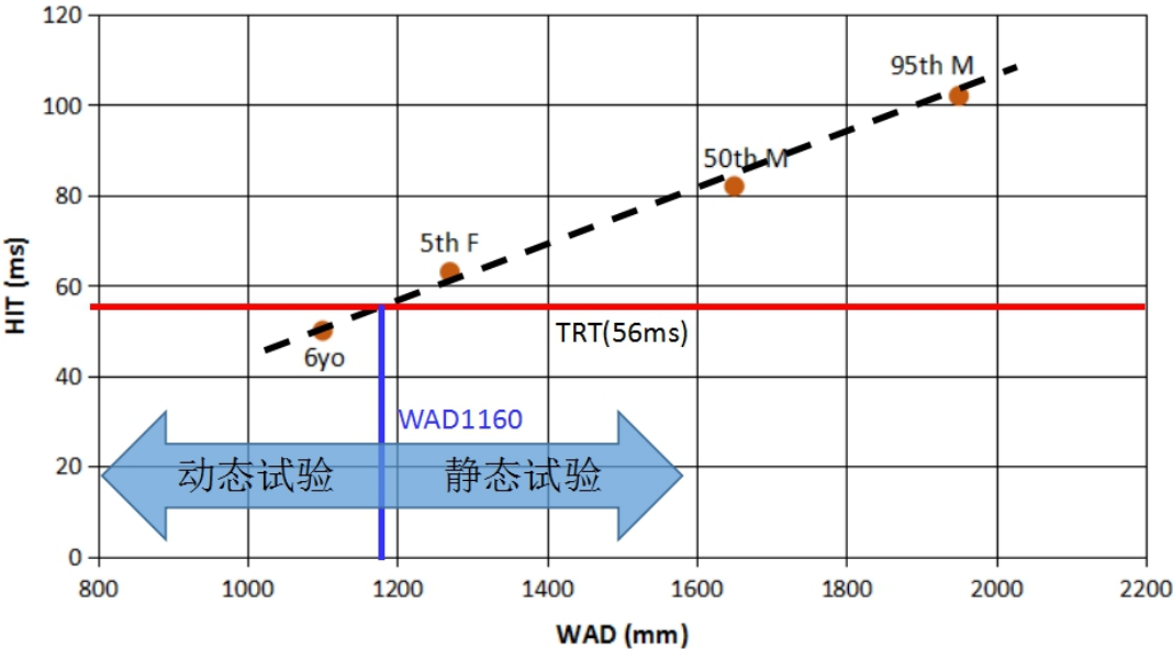
图 28 WAD vs HIT 关系图
