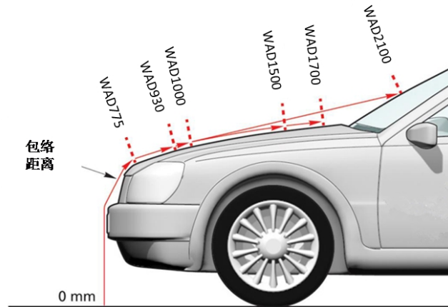
图 5 包络线的确定
