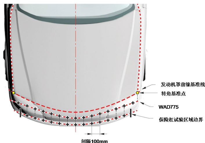
图 22 标记腿型试验区域网格点
