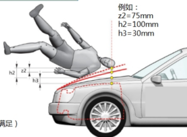
图 31 发动机罩变形要求
