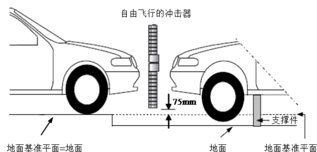
图 26 柔性腿型对保险杠试验
