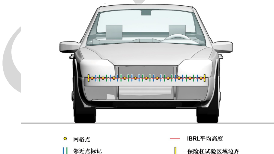
图 12 间距 100mm 的 IBRL 高度
