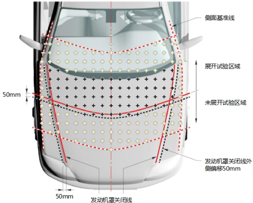
图 29 满足低起爆下限速度的区域
